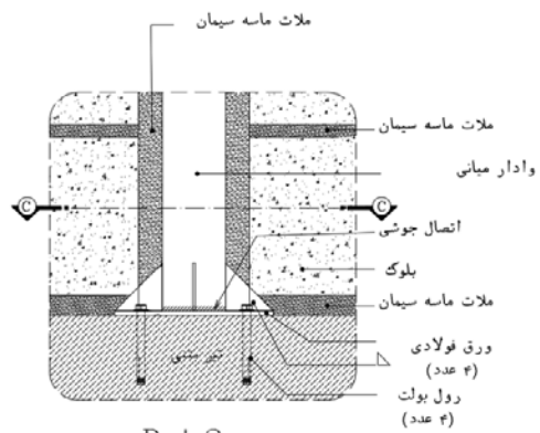
Det.2
