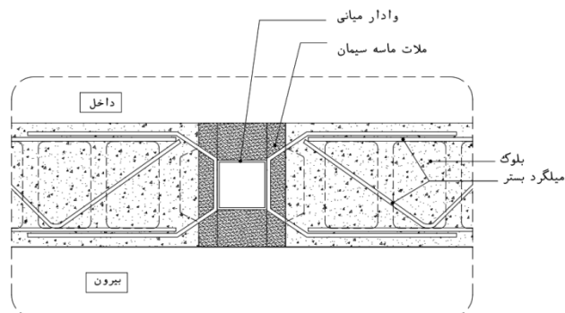
Det.3 sec.A-A
