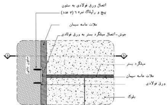
Det.1
